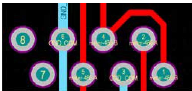
Порт лічильника
