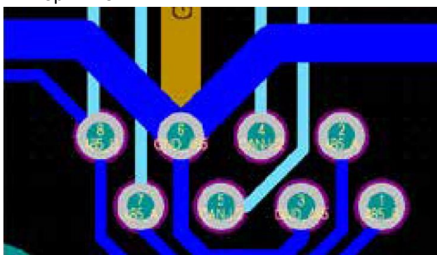
Порт BMS2
