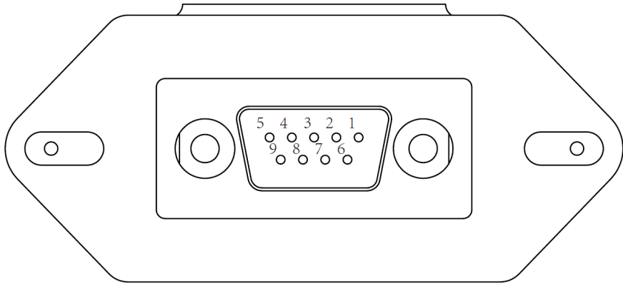
Wi-Fi/RS232
