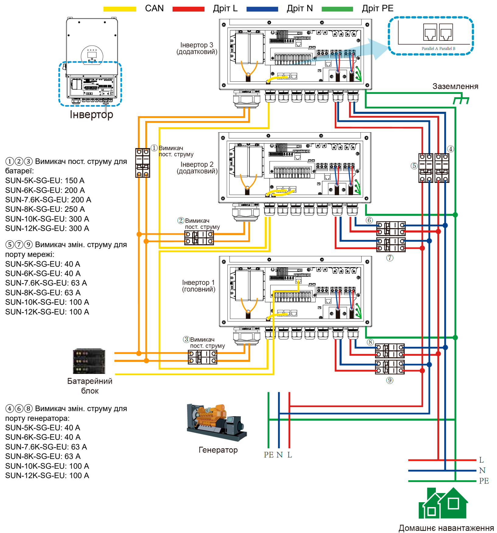
Головний інвертор
